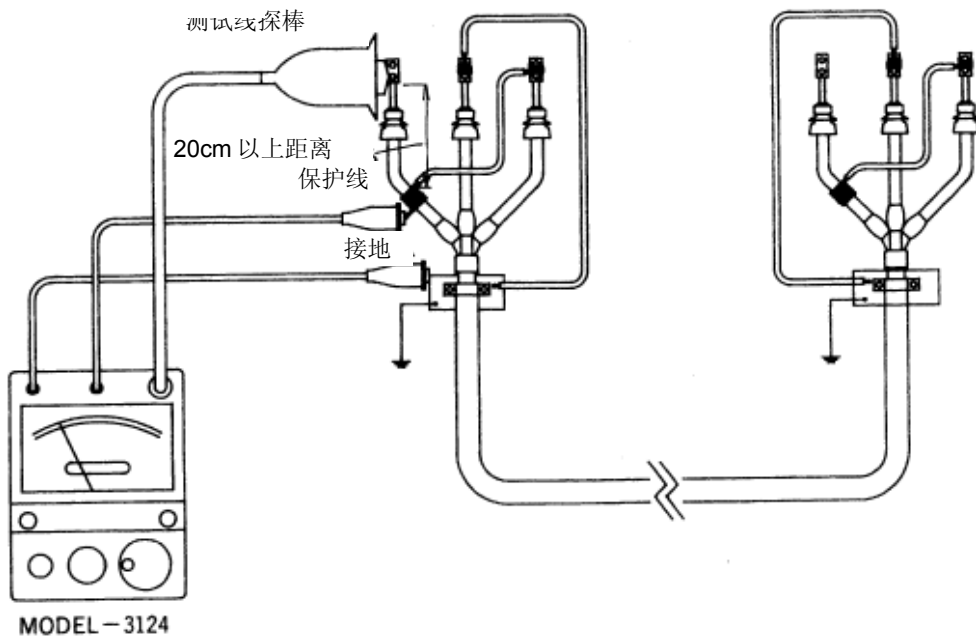
图 2 使用保护线
