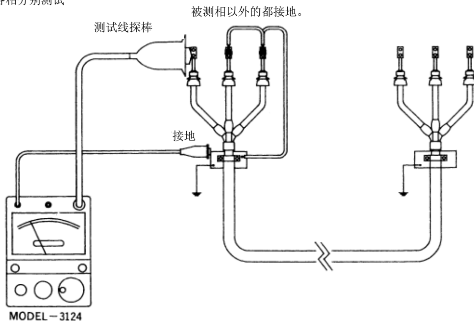
图 1 不使用保护线
